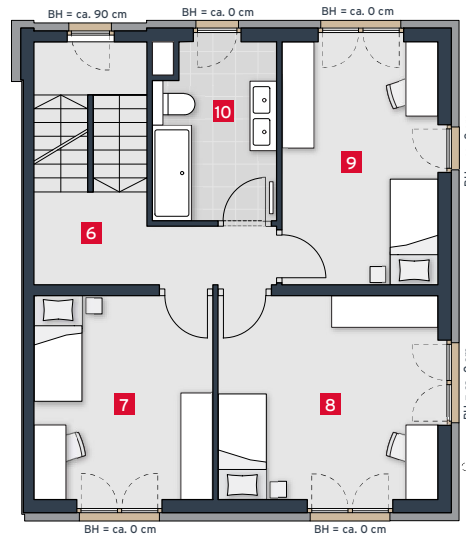
OBERGESCHOSS
