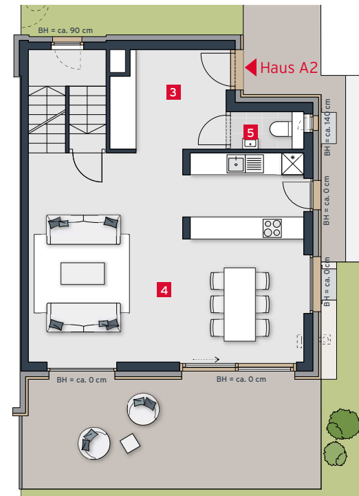
ERDGESCHOSS
