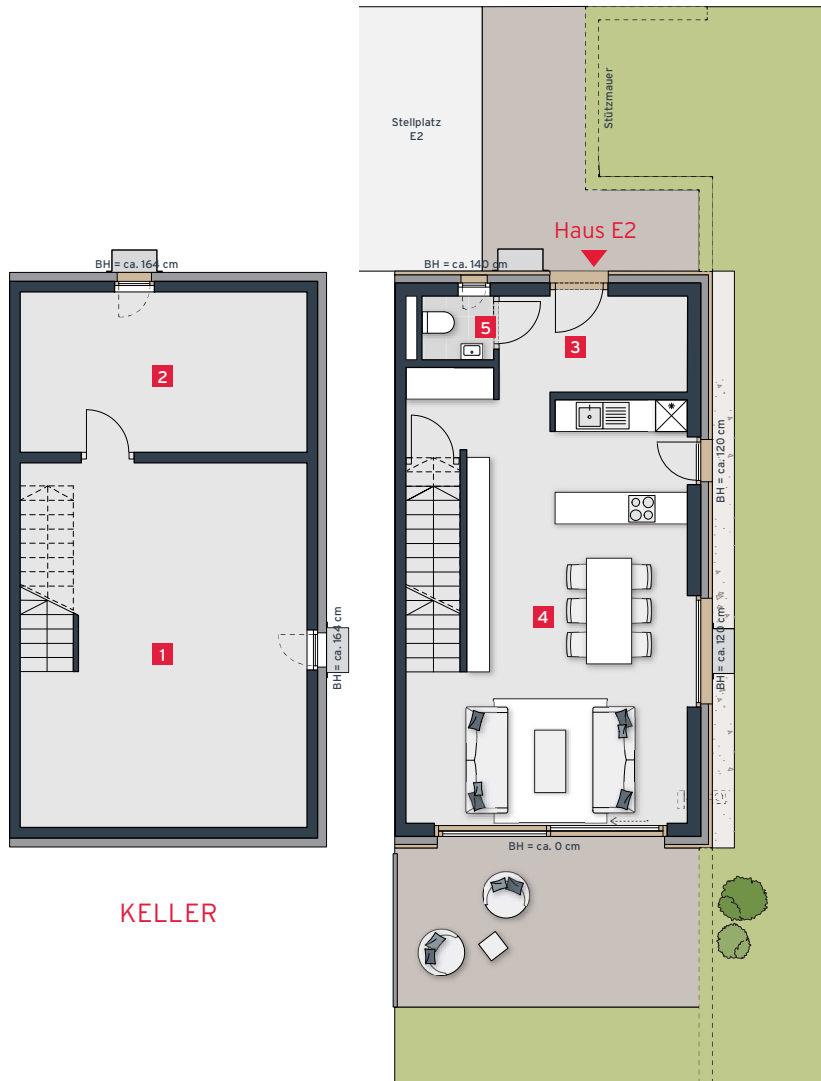
ERDGESCHOSS
