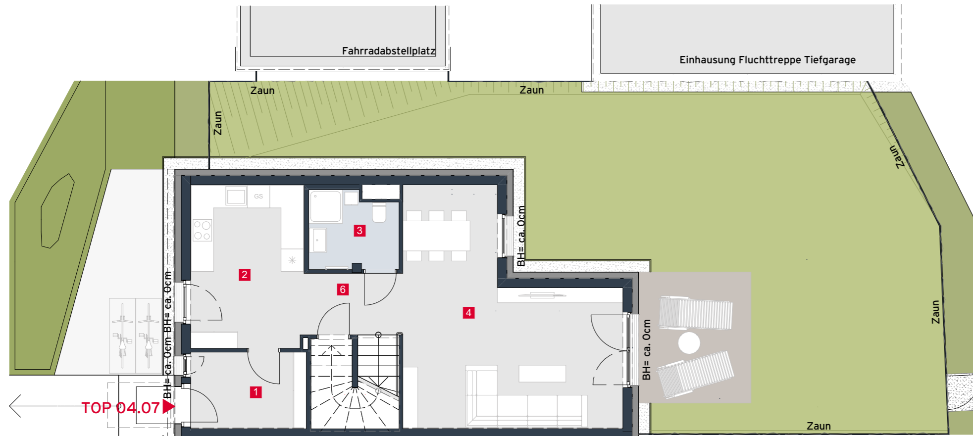
Erdgeschoss
