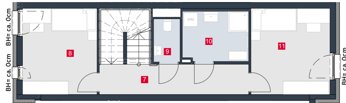
1. Obergeschoss
